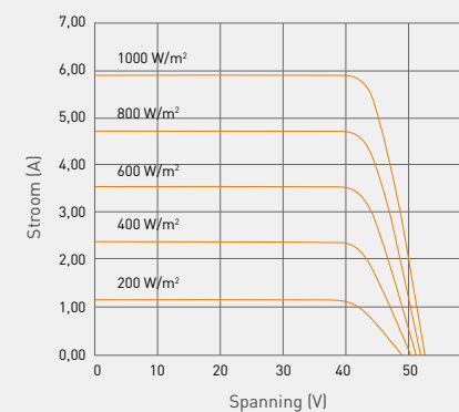
Referentiegegevens voor model VBHN245SJ25 (Celtemperatuur: 25 °C.)
