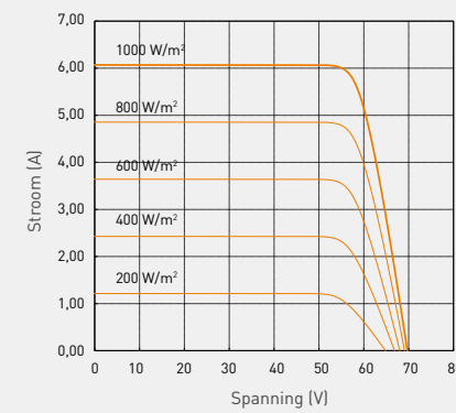
Referentiegegevens voor model VBHN330SJ47 (Celtemperatuur: 25 °C.)
