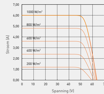
Referentiegegevens voor model VBHN295SJ46 (Celtemperatuur: 25 °C.)
