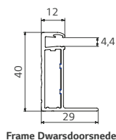
Frame Dwarsdoorsnede
