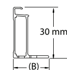
FRAMEPROFIEL
